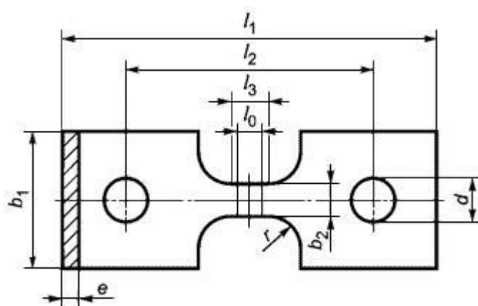
Рисунок 1 - Образец типа 3
