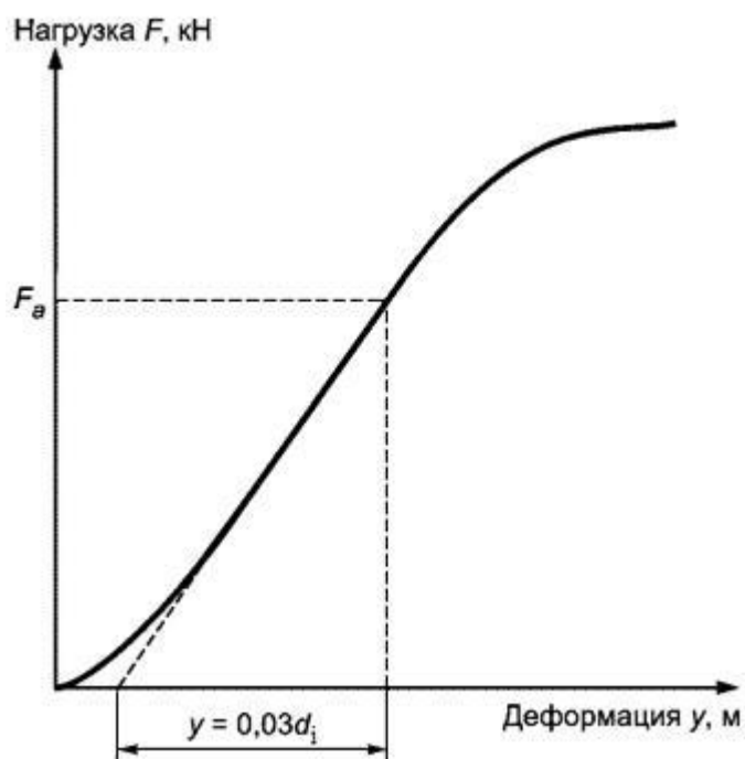
Рисунок В.1 - Кривая "нагрузка-деформация"
