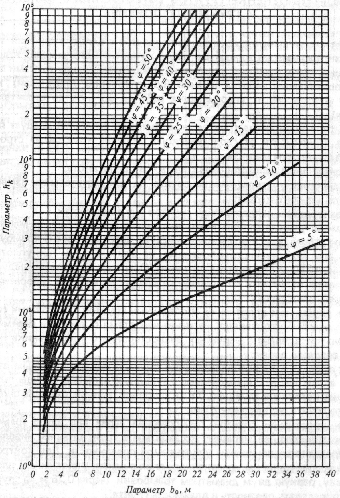
Черт. 6. Графики для определения параметра b_0
